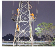
Các tổ, đội tăng cường kiểm tra phát hiện, xử lý những khiếm khuyết trên lưới điện. Trong ảnh: Điện lực Phú Bình sửa chữa lưới điện chống phát nhiệt.
